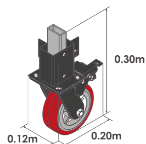
Ruedas 6" (4 unidades)
