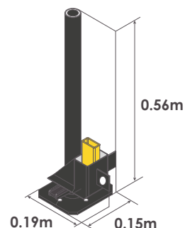
Nivelador (4 unidades)
